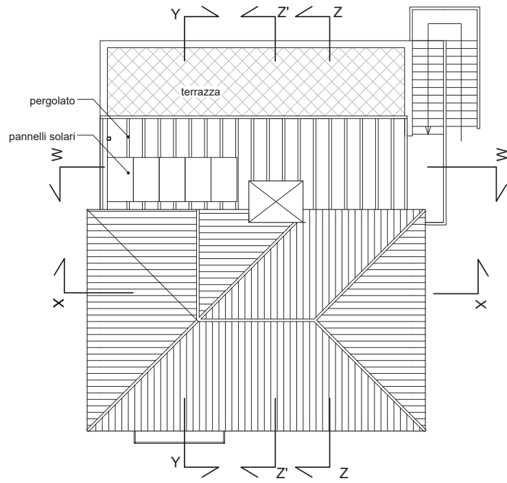
pianta della copertura
