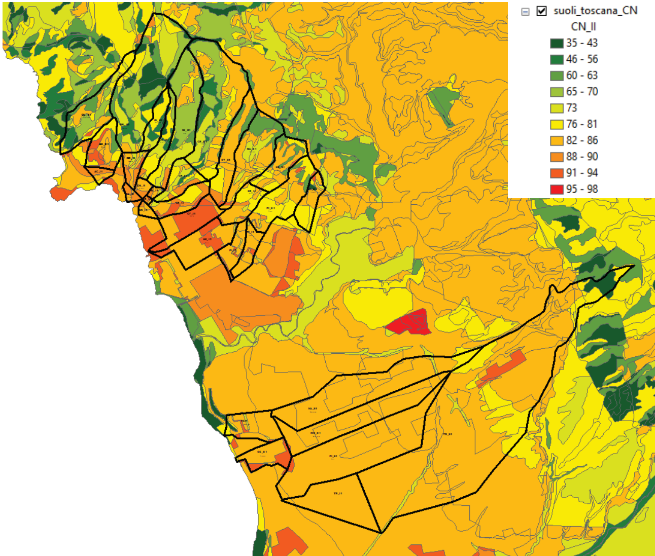
Figura 3-5: Andamento spaziale del parametro CN-II nell'area di interesse: la gradazione cromatica da verde a rosso indica aree rispettivamente da molto permeabili a sostanzialmente impermeabili. Le linee di colore nero indicano i bacini idrografici di interesse.
