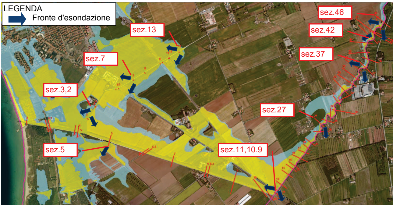
Figura 7-8: planimetria del fosso dei Fichi oggetto di studio con l'indicazione dei fronti di esondazione.
