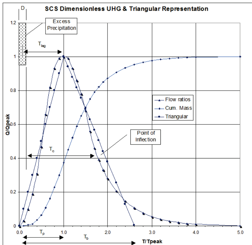
Figura 3-6: IUH-SCS
