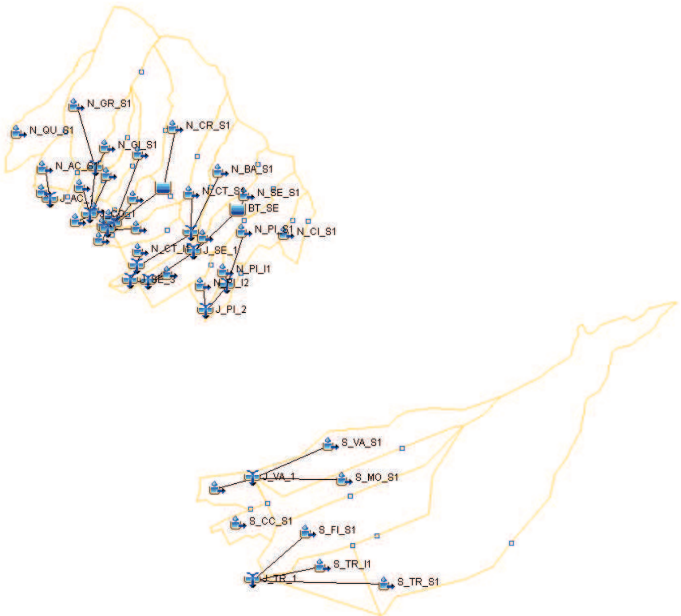
Figura 3-10: Modello idrologico semidistribuito implementato mediante il software HEC-HMS.
