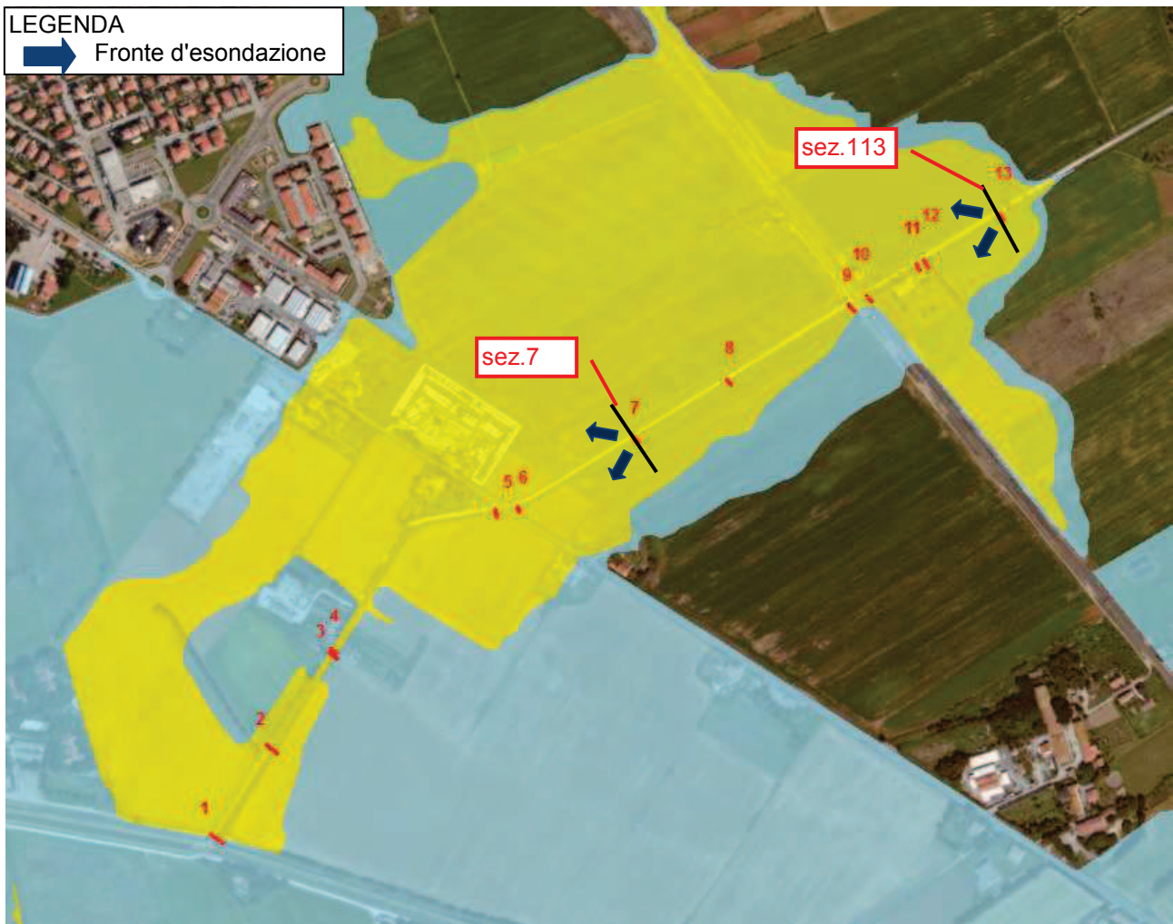
Figura 7-8: planimetria del fosso dei Fichi oggetto di studio con l'indicazione dei fronti di esondazione.
