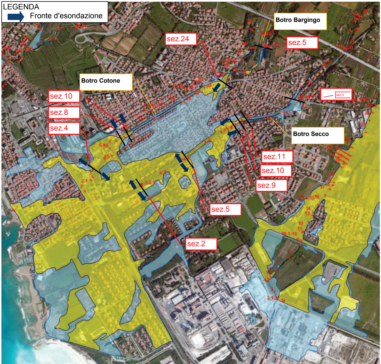
Figura 7-5: planimetria dei botri Cotone, Bargingo e Secco oggetto di studio con l'indicazione dei fronti di esondazione.
