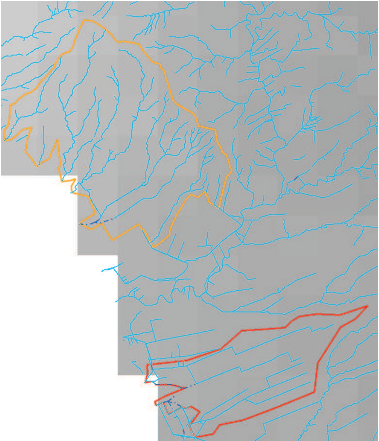
Figura 3-3: Individuazione delle porzioni Nord (perimetro arancio) e Sud (perimetro rosso) dei bacini idrografici e stima dei parametri delle LSPP a partire dai dati spaziali in formato raster forniti dalla Regione Toscana.
