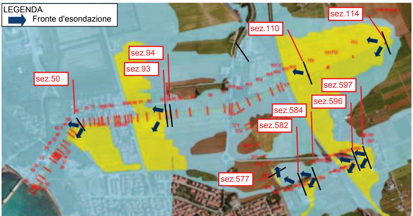
Figura 7-7: planimetria dei fossi Vallecorsa e Mozzicone oggetto di studio con l'indicazione dei fronti di esondazione.
