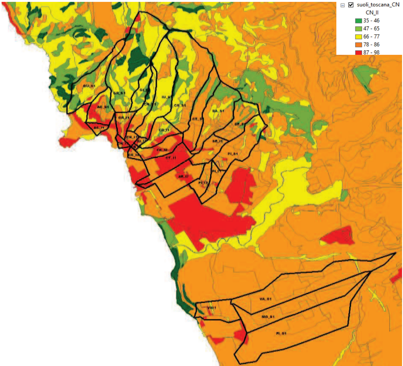
Figura 3-5: Andamento spaziale del parametro CN-II nell'area di interesse: la gradazione cromatica da verde a rosso indica aree rispettivamente da molto permeabili a sostanzialmente impermeabili. Le linee di colore nero indicano i bacini idrografici di interesse.
