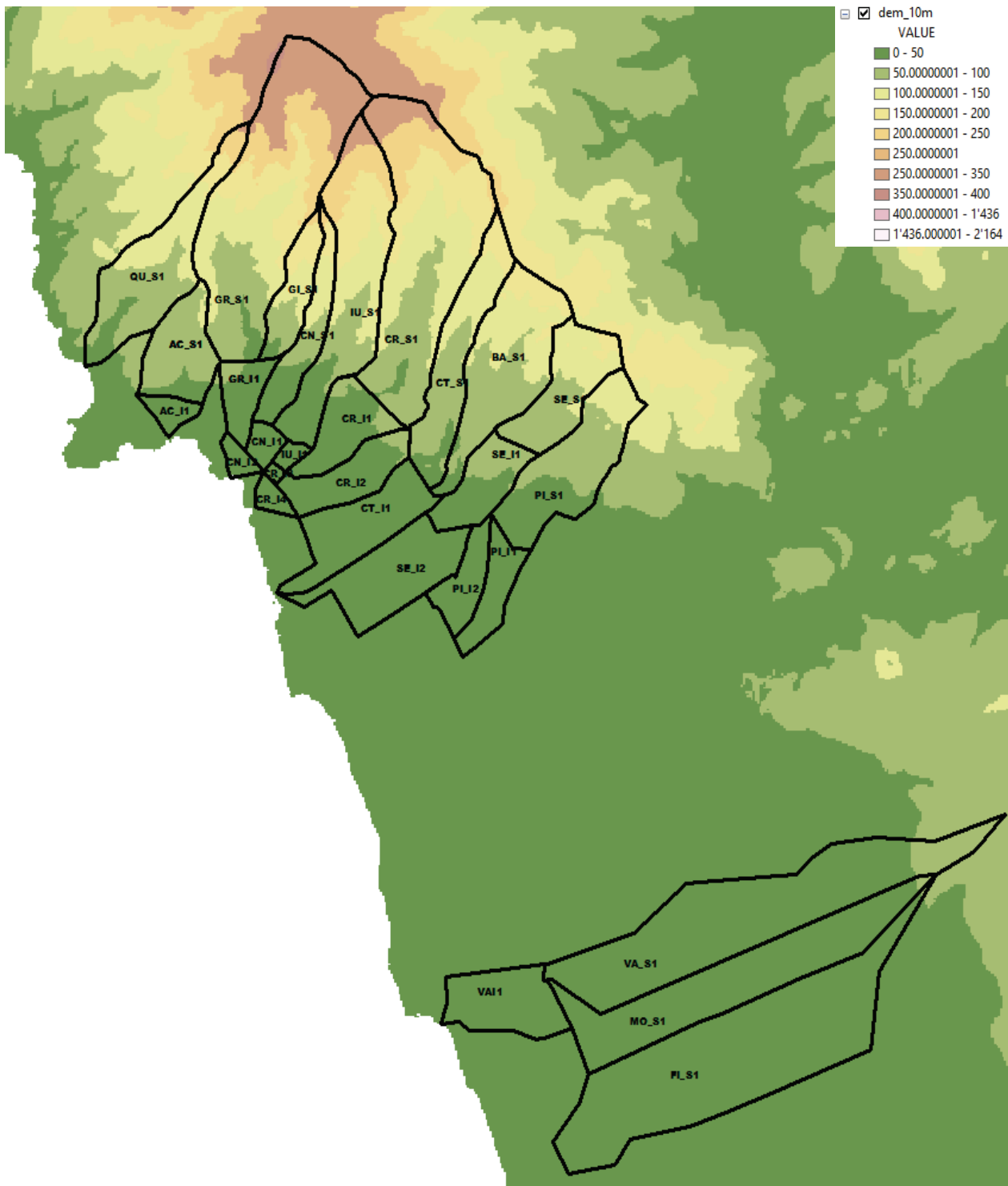
Figura 3-9: Morfologia del territorio di interesse.
