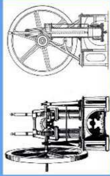
il motore di Barsanti e Matteucci - 1853
